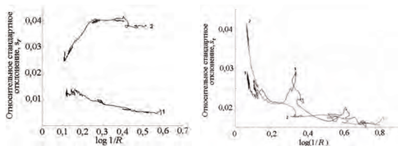
Зависимости стандартного относительного отклонения от интенсивности спектров рассыпных (слева) и таблетированных (справа) кормов
