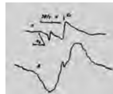
Рис. 3. Спектры ЭПР замороженных растворов хлора в фторбензоле (а) и гексафторбензоле (б) после фотолиза в ближнем УФ. (а) дополнительно показана сверхтонкая структура спектра, связанная с расщеплением на атоме фтора [7,8].
