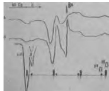
Рис. 2. Спектры ЭПР замороженных растворов хлора в толуоле (а) и дейтеротолуоле (б) после фотолиза. Внизу с увеличением показана изотопная структура линий, связанная с различием ядерного магнитного момента для изотопов Cl^{35} и Cl^{37} [7].
