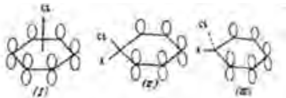
Рис. 1. Возможные структуры комплексов атомов хлора с ароматическими соединениями [7, 8].
