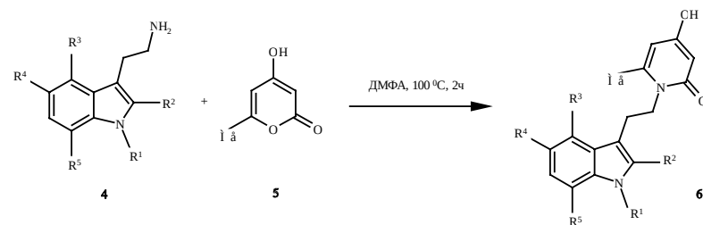
Схема 2. Синтез пиридонотриптамина 6
