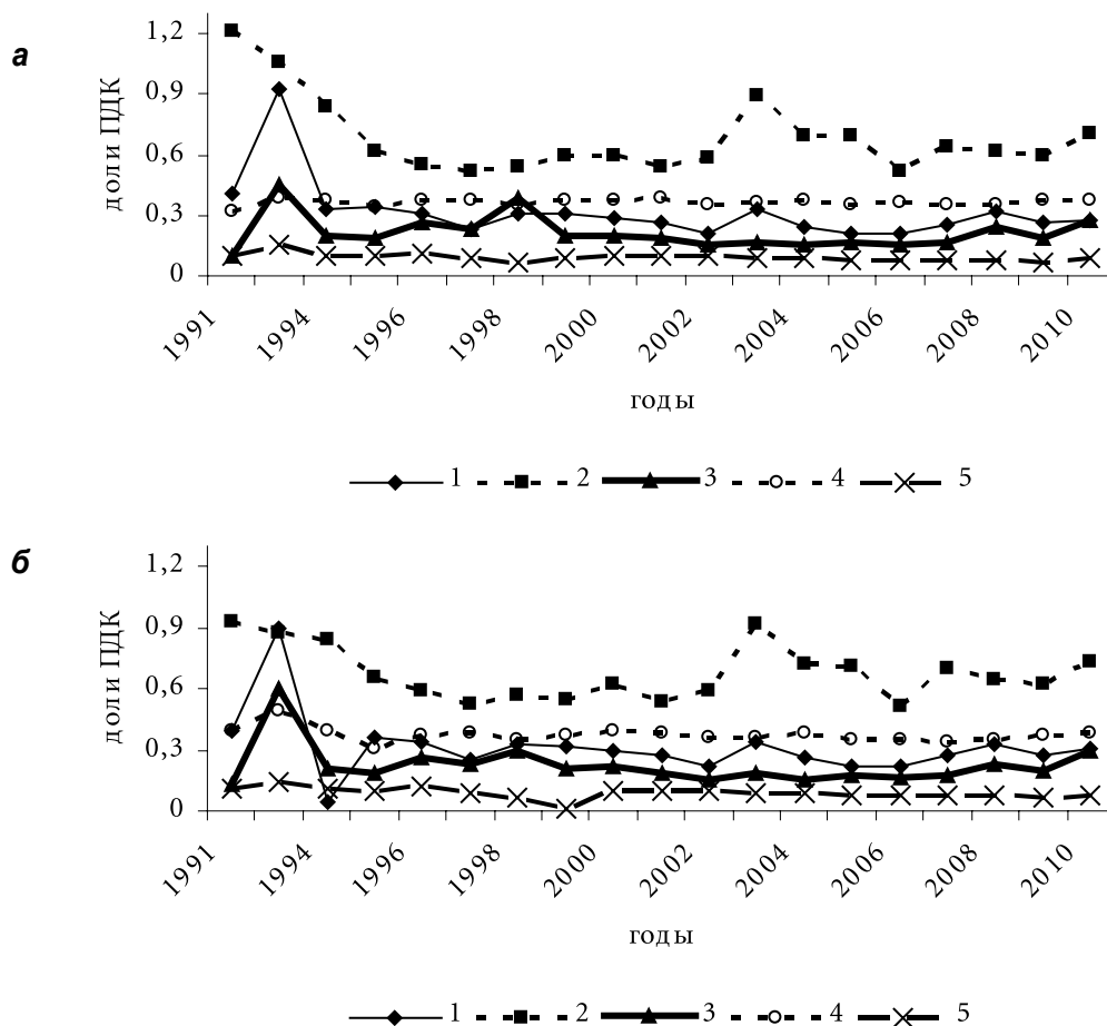
Рис. 2. Динамика гидрохимических показателей Днестра выше (а) и ниже (б) по течению от очистных сооружений г. Рыбница: ХПК (1), БПК 5 (2), аммиак (3), сухой остаток (4), хлориды (5)
