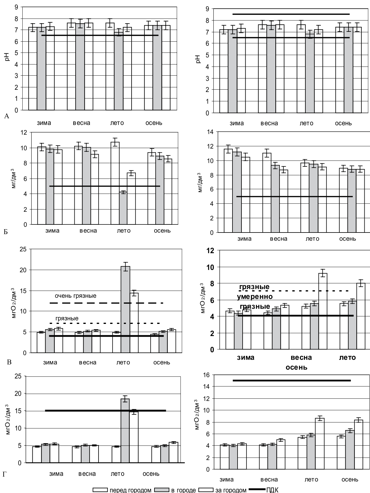
Рис.1. Сезонная динамика показателей pH (А), растворенного кислорода (Б), БПК 5 (В) и перманганатной окисляемости воды из р. Серет в акватории г. Чертов в 2008-2009 гг.
