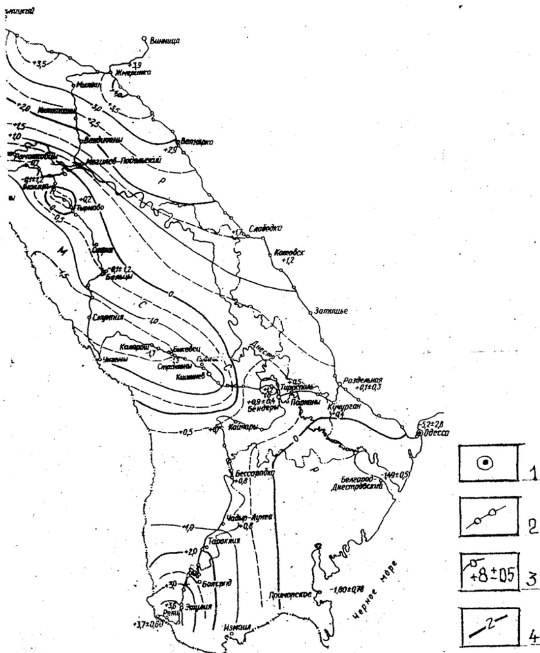
Рис. 1. Карта современных вертикальных движений земной коры Молдовы и западной части Украины: 1 – уровеньный пункт; 2 – линии повторного нивелирования; 3 – пункты с абсолютными значениями скоростей и ошибками их определения (мм/год); 4 – изолинии скорости (мм/год)
