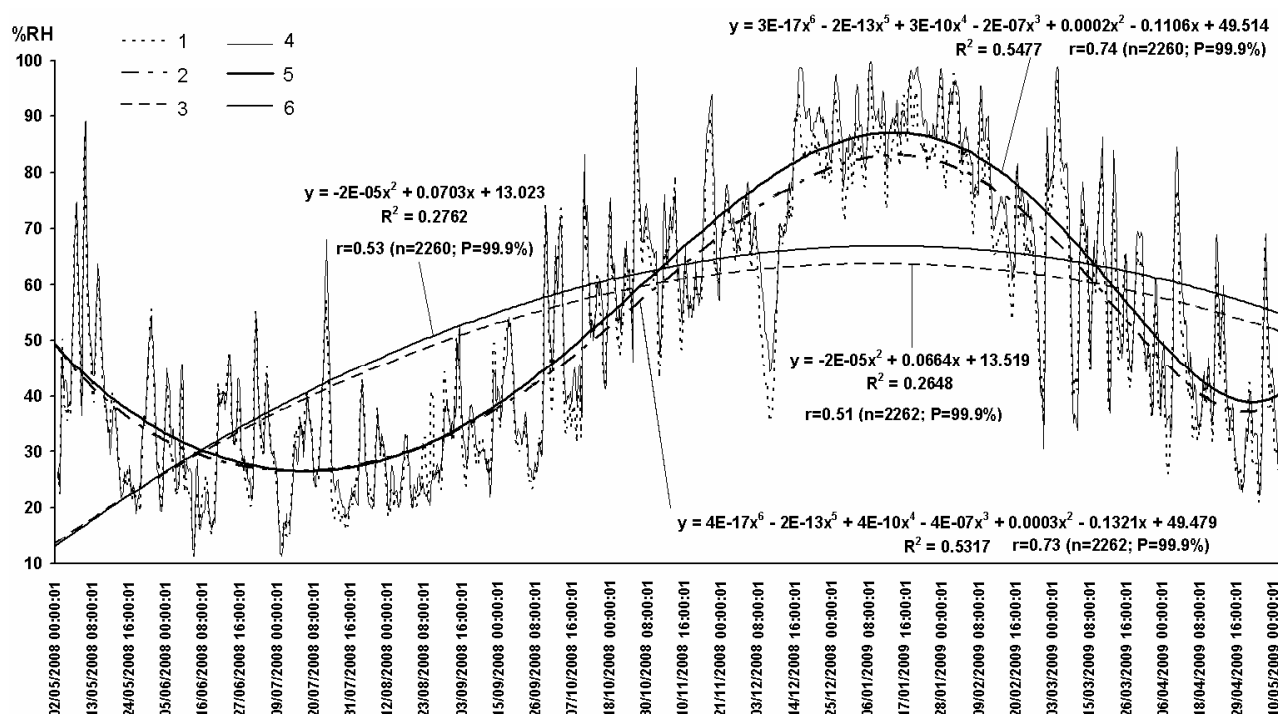
Рис. 2. Сравнение кривых относительной влажности воздуха (в %) ежедневного осреднения (скользящих средних 6 периода) и полиномиальных трендов (второго и шестого порядка) на участке без растительности в Муйнаке (кривые 1, 2, 3) и на контрольном участке (без полива) в посадках саксаула Haloxylon aphyllum на обсохшем дне Аральского моря (кривые 4, 5, 6) в период со 02 мая 2008 года по 10 мая 2009 года. Fig. 2. Comparison of curves of daily averaging trend-line (6-period Moving Average) and polynomial trend-lines of relative humidity of air in % on plots without vegetation in Muynak (curves 1, 2, 3) and on an index plot with a vegetation Haloxylon aphyllum (curves 4, 5, 6) in a period from May, 02 nd , 2008 till May, 10 nd , 2009.
