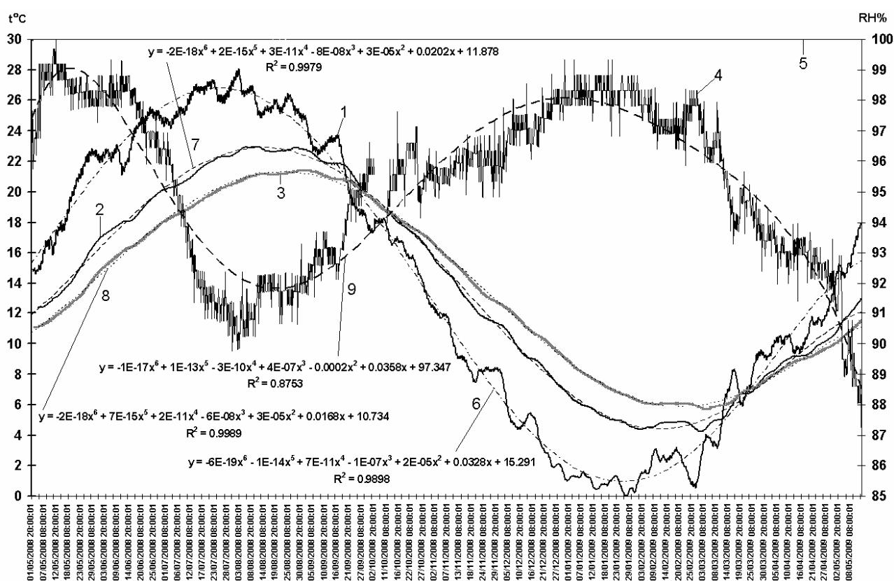
Рис. 3. Сравнение температуры почвы ( t^{\circ}\text{C} ) разных горизонтов (40 см, 100 см и 150 см – кривые 1, 2, 3 соответственно) и относительной (RH%) влажности воздуха в порах почвы (40 см, 100 см – кривые 4 и 5) в контрольном разрезе № 2 на участке солончаков с посадками саксаула ( Haloxylon aphyllum ) без полива по данным прибора-регистратора за период со 02 мая 2008 года по 10 мая 2009 года: кривые 1, 2, 3, 4, 5 – фактические измерения; кривые 6, 7, 8, 9 – полиномиальные тренды.
