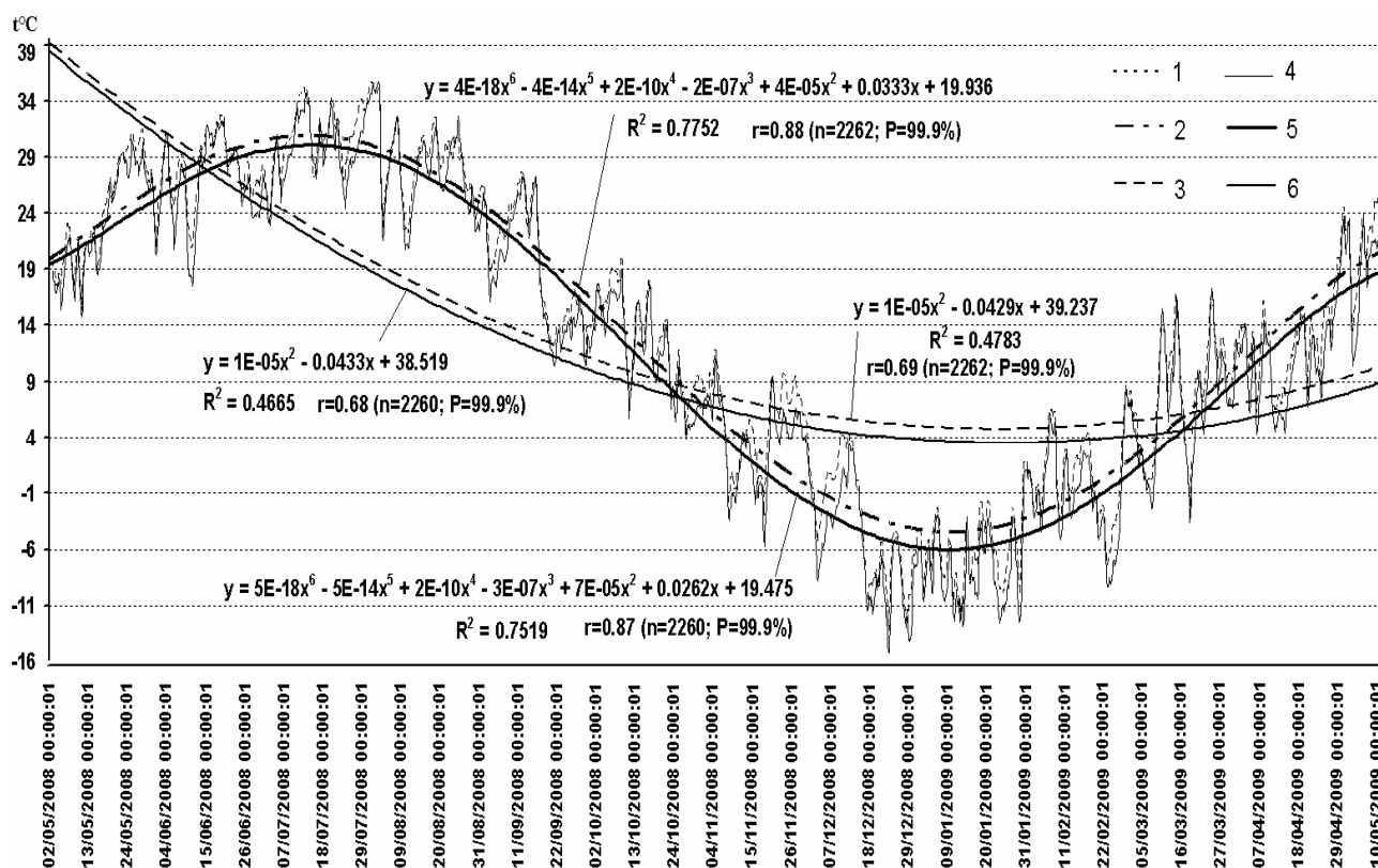
Рис. 1. Сравнение кривых температуры воздуха ( t^{\circ}\text{C} ) ежедневного осреднения (скользящих средних 6 периода) и полиномиальных трендов (второго и шестого порядка) на участках без растительности в Муйнаке (кривые 1, 2, 3) и на контрольном участке (без полива) в посадках саксаула Haloxylon aphyllum на обсохшем дне Аральского моря (кривые 4, 5, 6) в период со 02 мая 2008 года по 10 мая 2009 года (на рисунках 1, 2 и 3 – осреднение по данным ежедневных измерений через каждые 4 часа). Fig. 1. Comparison of curves of daily averaging trend-line (6-period Moving Average) and polynomial trend-lines temperatures of air ( t^{\circ}\text{C} ) on plots without vegetation (curves 1, 2, 3) and on key site with vegetation Haloxylon aphyllum (curves 4, 5, 6) in a period from May, 02 nd , 2008 till May, 10 nd , 2009 (In a figures 1, 2 and 3 – averaging trendline till the data of daily measurements in each 4 hours).
