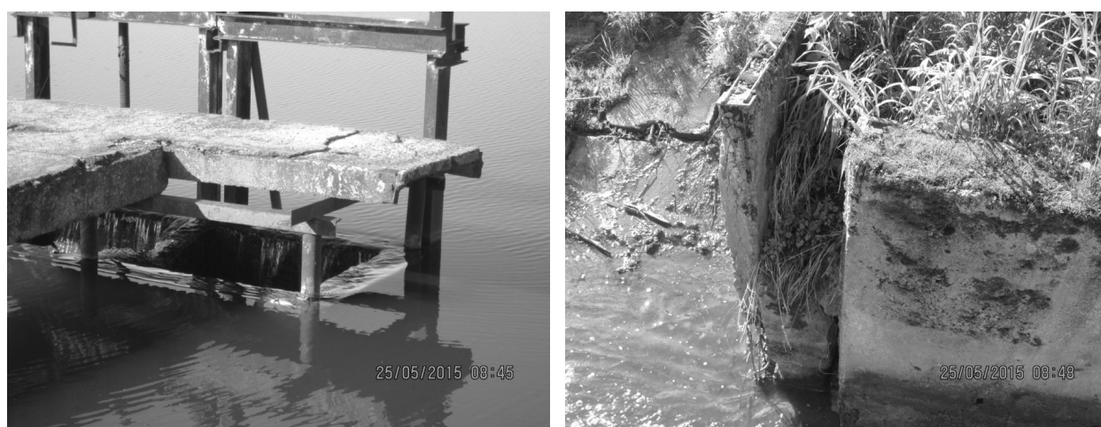
Рис. 2. Техническое состояние ГТС пруда-накопителя у д. Кузевичи
