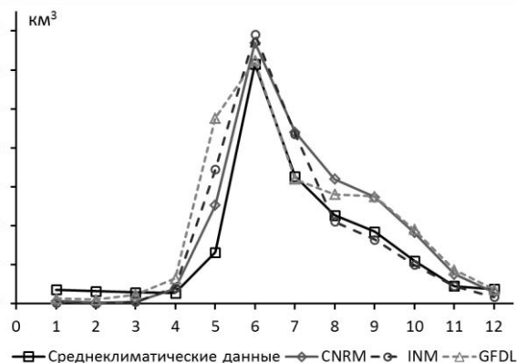
Рис. 2. Среднеклиматические гидрографы притока пресной воды в СЛО
