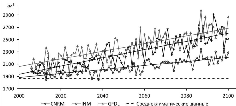
Рис. 3. Межгодовая изменчивость общего стока сибирских рек в СЛО в XXI веке. Сплошной линией представлен линейный тренд стока, пунктирной линией - климатическое значение
