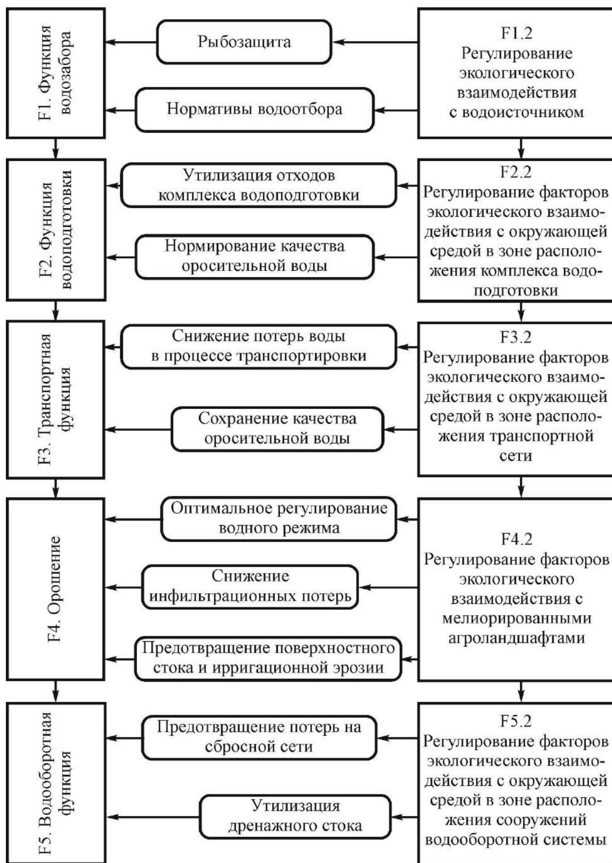
Рисунок 1 – Компонентно-функциональная модель оросительной системы. Экологическая функция
