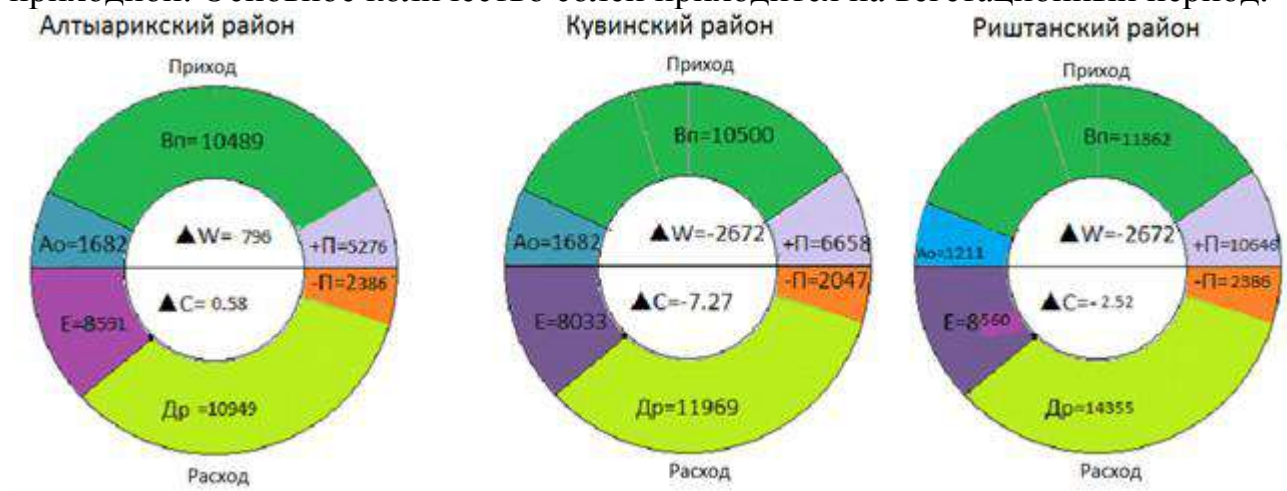
Рис 3. Диаграмма общего водно-солевого баланса по Алтыарикскому, Кувинскому и Риштанскому району Ферганской области. A o -атмосферные осадки, V o -вододача, E -суммарное испарение, Др -дренажный сток, +П -подземный приток, -П -подземный отток, ▲W и ▲C -общие изменения запасов влаги и солей на балансовой площади.
