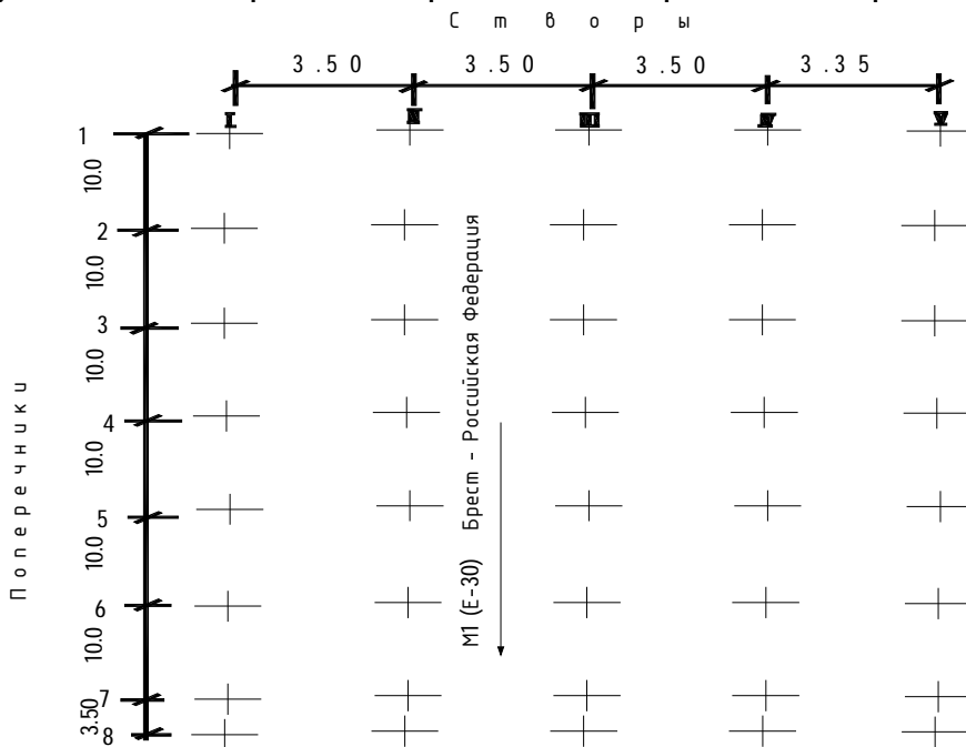
Рисунок 1 – Схема разбивки пикетажа
