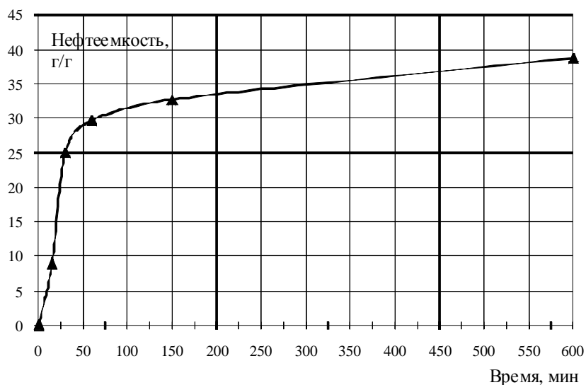
Рисунок – Кинетика поглощения нефти сорбентом «Ливсор-С»
