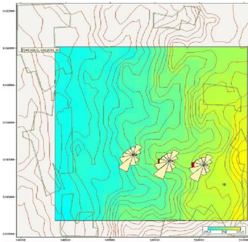
Рисунок – Оцифрованный рельеф, эффекты экранирования ветроустановок, скорость ветра и шероховатость поверхности на площадке д. Жиличи
