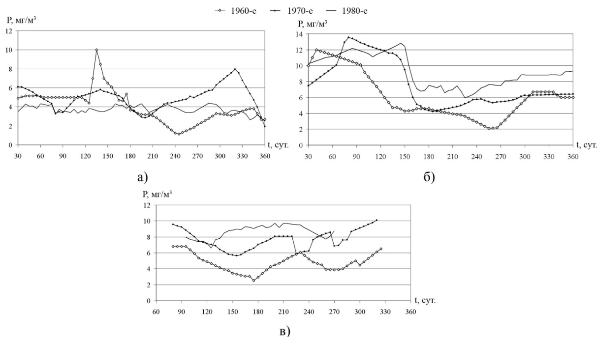
Рис. 7. Динамика средних концентраций P-PO_4 мгP/м³ для 1960, 70 и 80-х гг. по створу: а – Базаиха, б – Лесосибирск, в – Игарка
