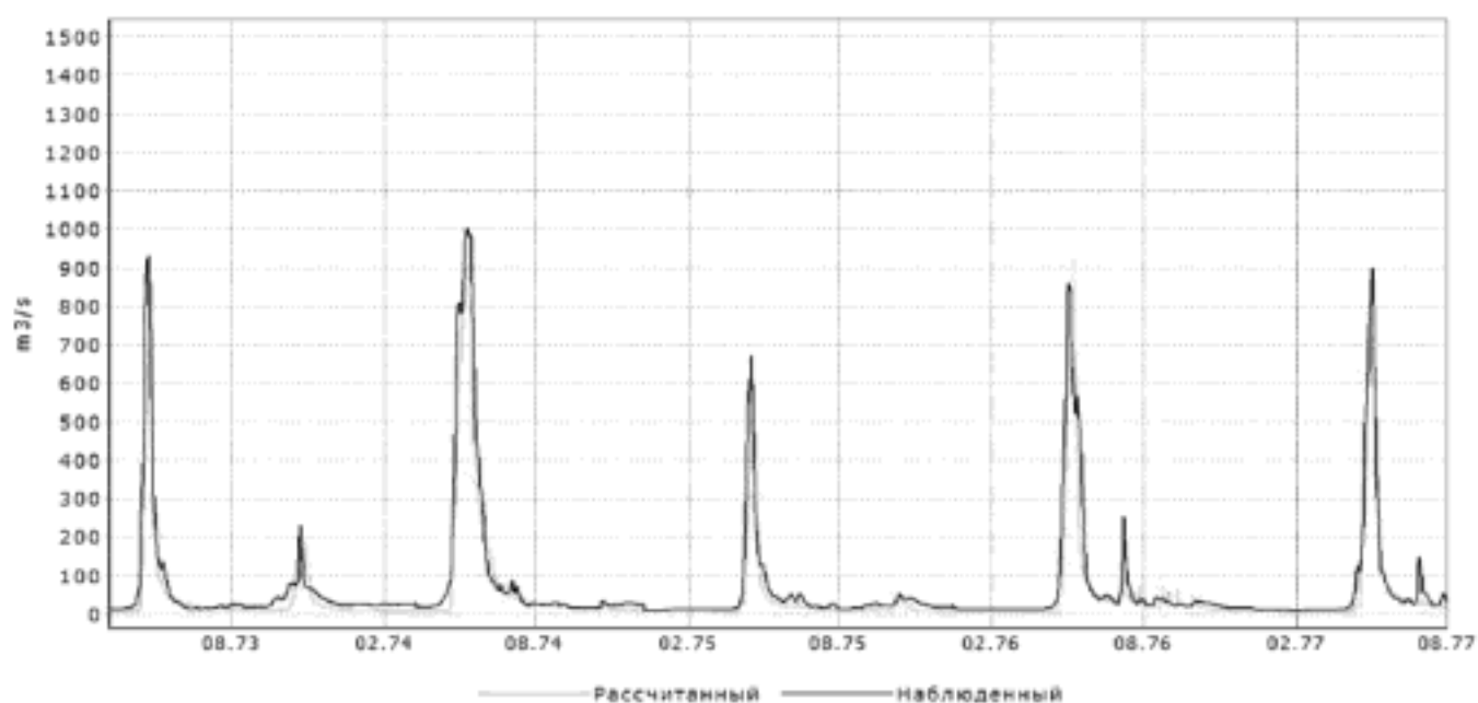
Рис.9. Гидрограф р. Камы (п. Волосническое)
