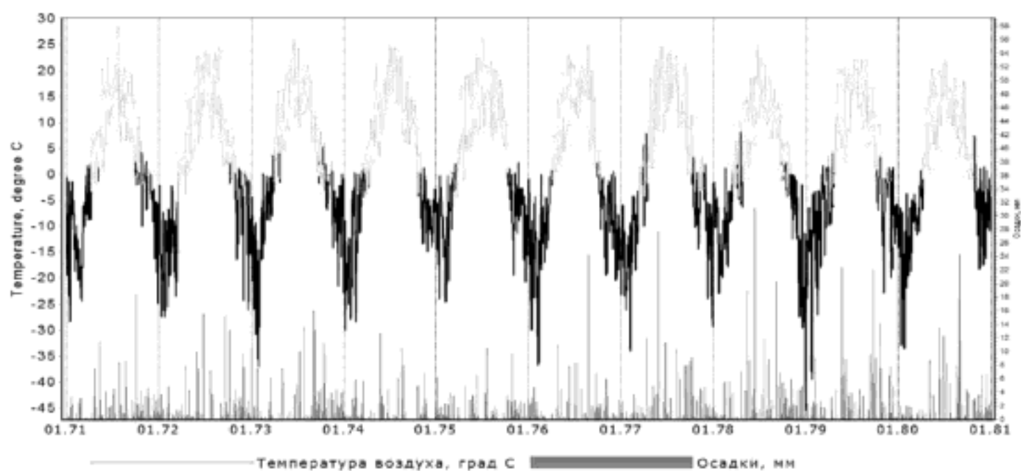
Рис.6. Графики исходной метеорологической информации по ст. Пермь
