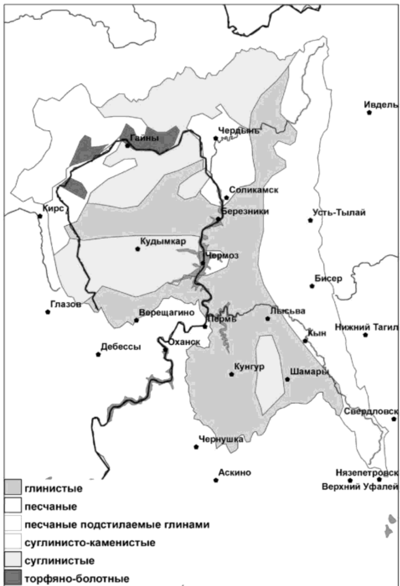
Рис. 2. Механический состав почвы бассейна Камского водохранилища [5]
