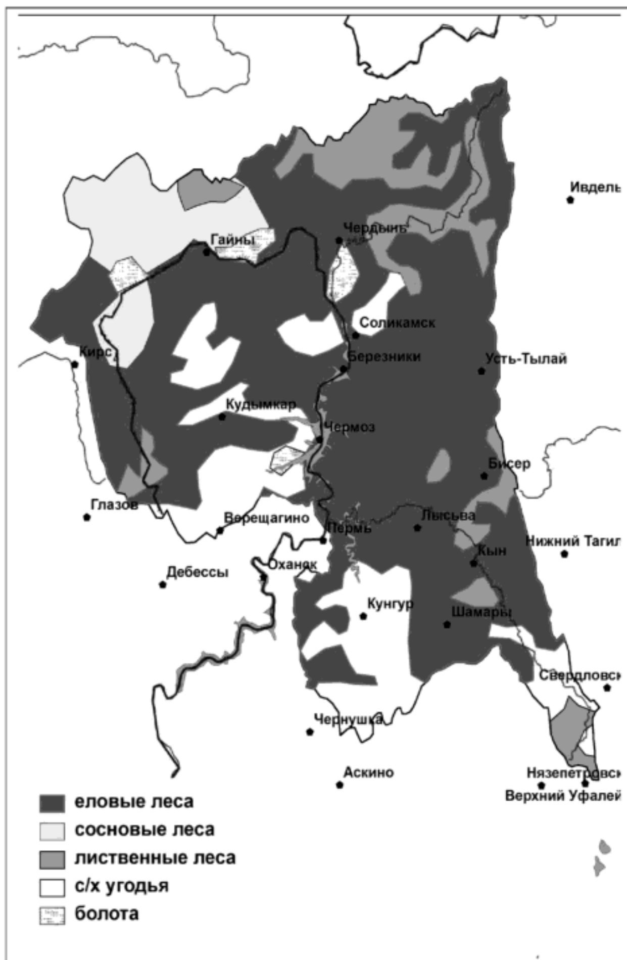
Рис. 3. Растительность бассейна Камского водохранилища [5]
