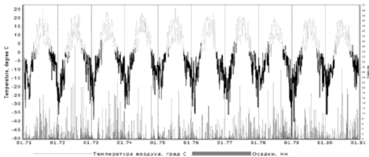
Рис.5. График исходной метеорологической информации по ст. Бисер
