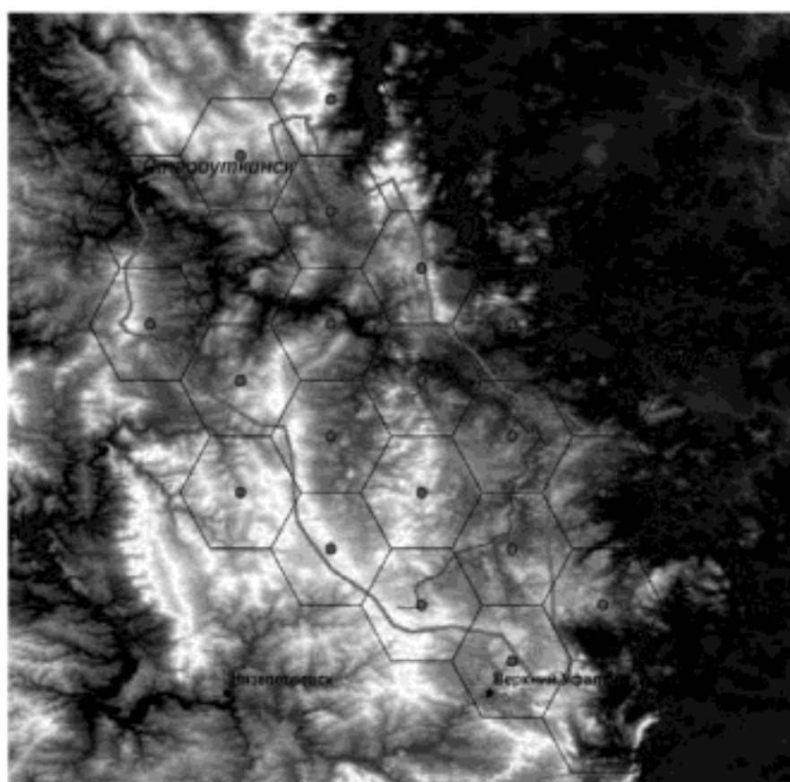
Рис. 1. Назначение РТ в бассейне р. Чусовой (п. Староуткинский)
