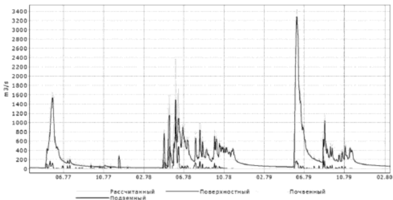
Рис. 12. Гидрографы стока по РСР на р. Чусовая (п. Лямино)
