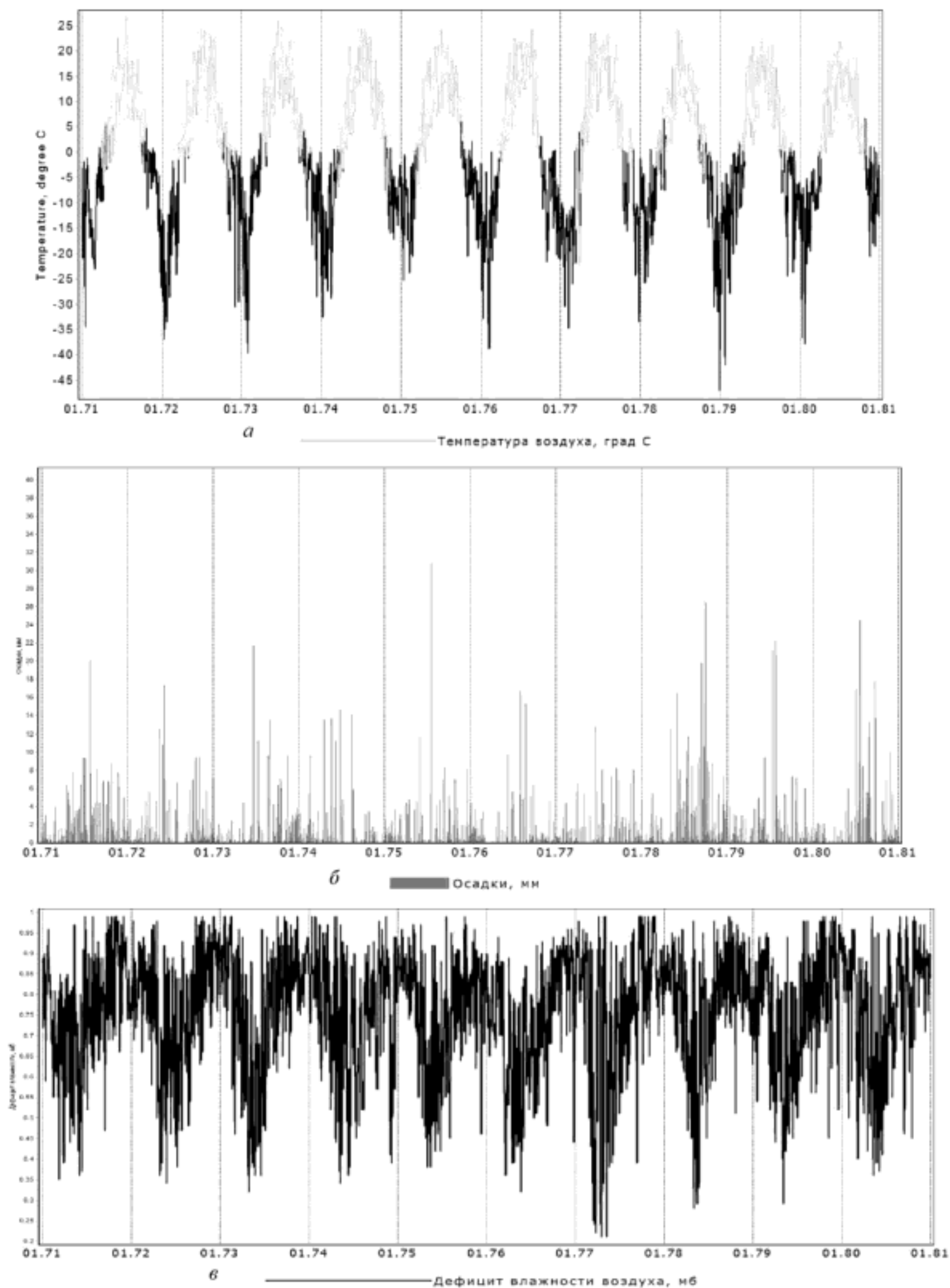
Рис. 4. Графики исходной метеорологической информации по г. Березники: а – температура воздуха, °С; б – осадки, мм; в – дефицит влажности воздуха, мбар.
