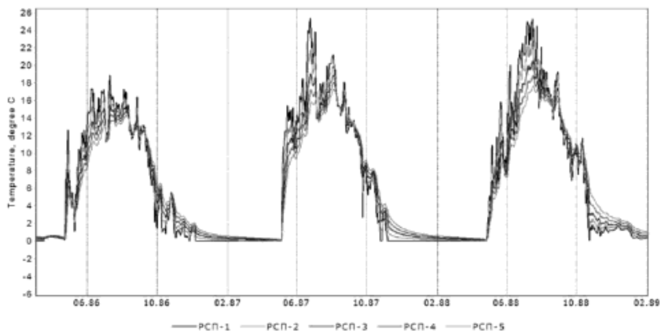
Рис. 8. Распределение температуры почвы по РСП (р.Чусовая–п. Лямино)
