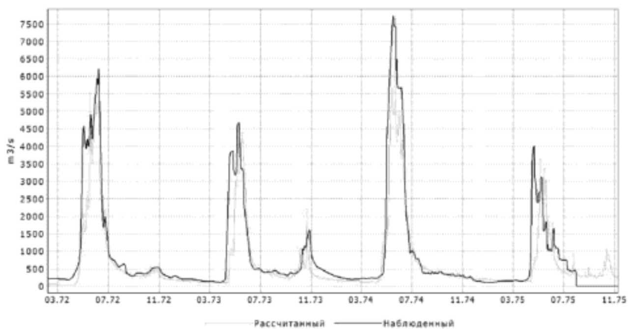
Рис. 10. Гидрограф р. Камы (п. Тюлькино)
