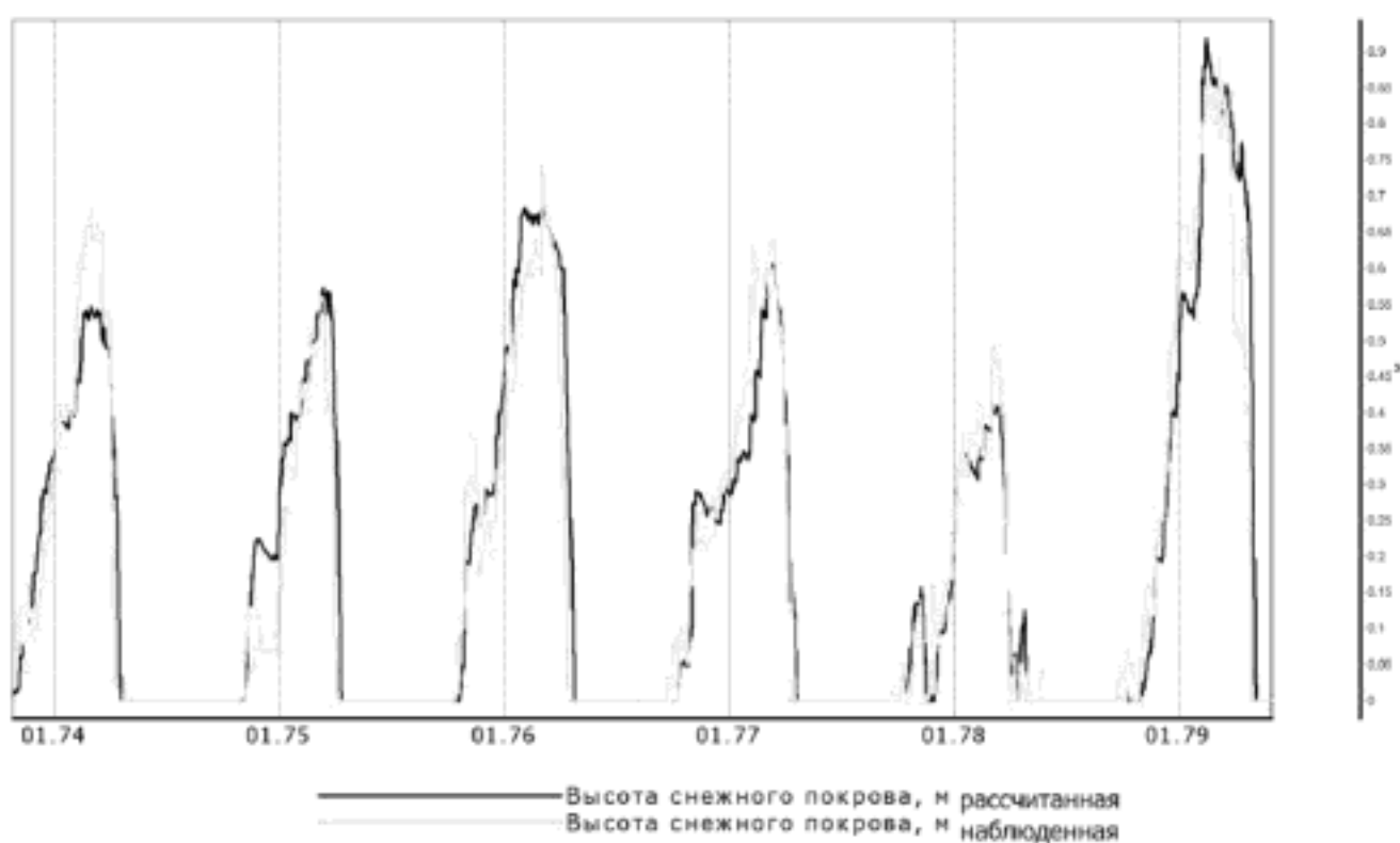
Рис. 7. Высота снежного покрова (р. Чусовая–п. Лямино)
